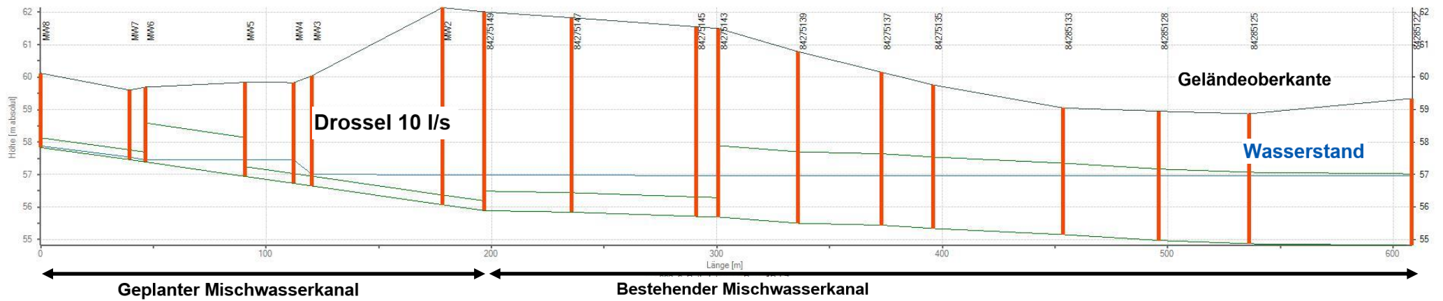
Abb. 1 -1: Längsschnitt Mischwasserkanal – eindimensionale Kanalnetzrechnung für Langzeitserie mit der Regenreihe Kläranlage Troisdorf Mülleken
