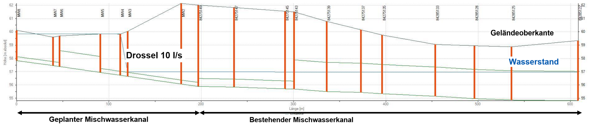
Abb. 1-2: Längsschnitt Mischwasserkanal – Gekoppelte Starkregenbetrachtung für ein 100-jährliches Niederschlagsereignis
